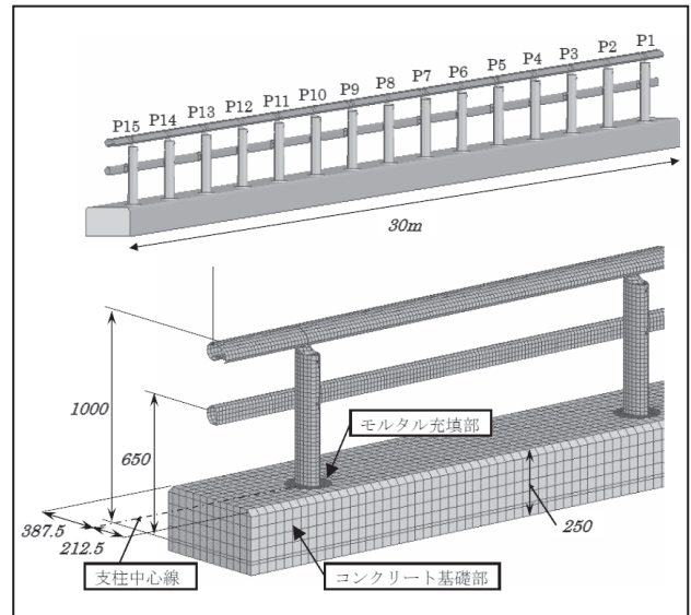
図-20 シミュレーションで用いた防護柵モデル
