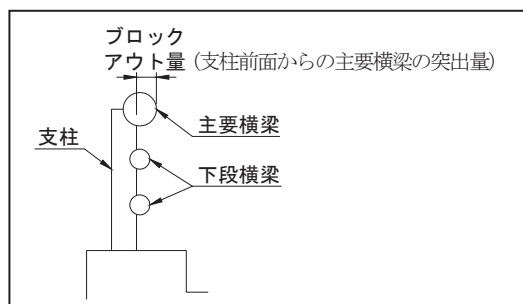
図-2 橋梁用防護柵の主要部材構成
