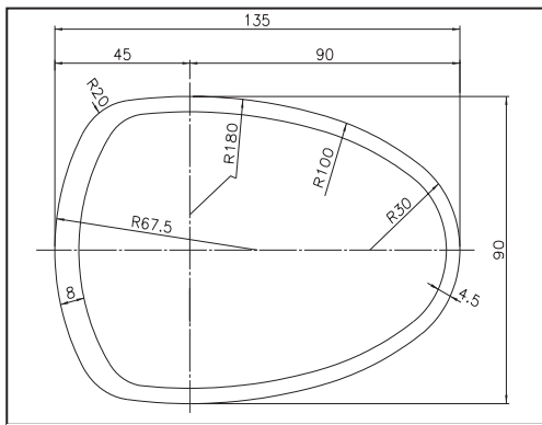
図-6 支柱のデザイン検討結果(断面図 単位はmm)
