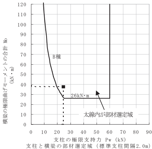
図-19 3本ビームタイプの部材選定域
