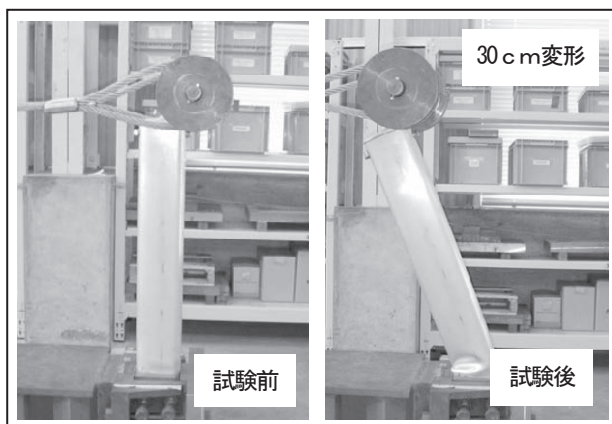
図-15 静荷重試験の状況
