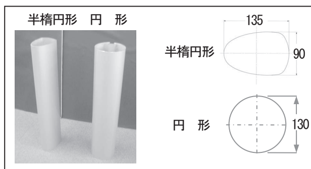
図-4 支柱形状の比較（半楕円形と円形）
