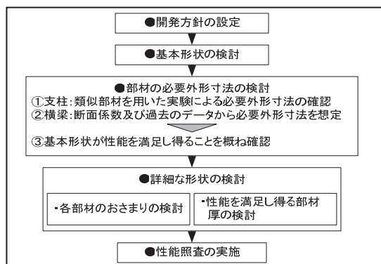
図-3 今回の防護柵開発の流れ
