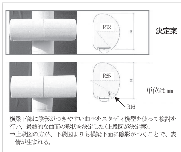
図-9 下段横梁の形状検討(3本ビームタイプの場合)
