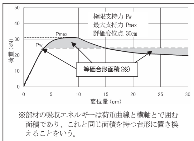
図-16 支柱の荷重～変位曲線 (供試体 No. 1 P_w=24.4 kN P_{max}=31.1 )
