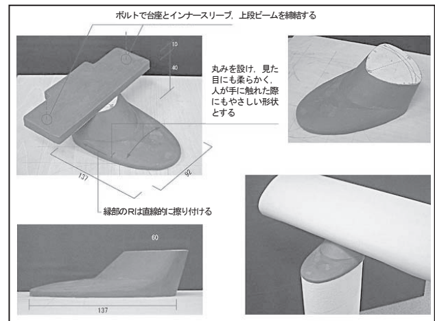
図-11 模型によるブラケットの形状検討
