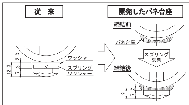
図-12 パネ台座検討図
