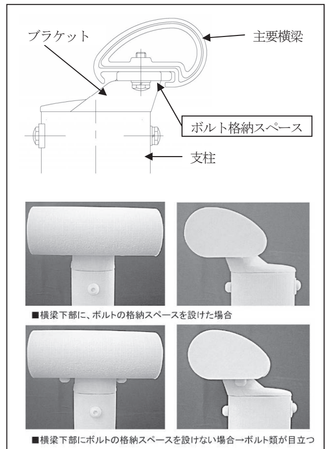
図-7 主要横梁の形状検討
