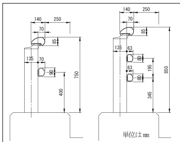
図-13 本防護柵の一般図 (左：2本ビームタイプ、右：3本ビームタイプ)
