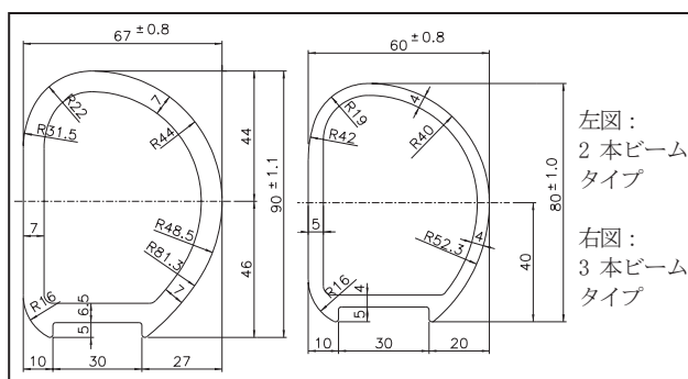
図-10 下段横梁のデザイン検討結果(断面図 単位はmm)
