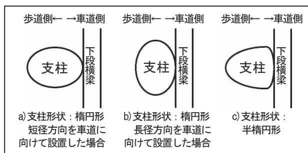
図-5 楕円形を基本とした支柱断面形状の比較検討
