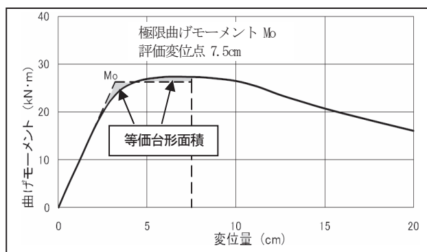
図-17 主要横梁の曲げモーメント変位曲線 (供試体 No. 1 M_o=26.3 kN・m)
