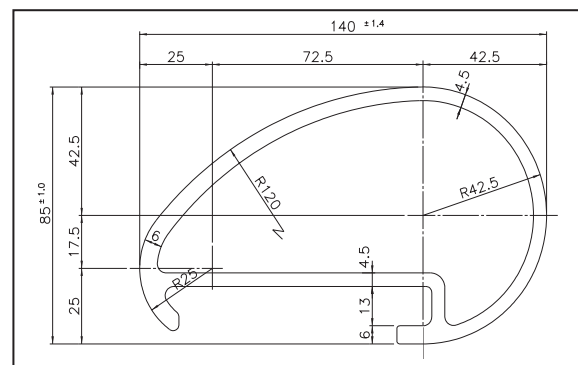
図-8 主要横梁のデザイン検討結果(断面図 単位はmm)
