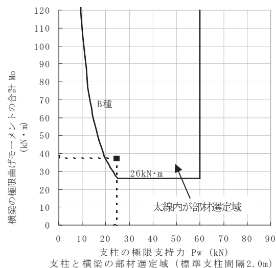
図-18 2本ビームタイプの部材選定域
